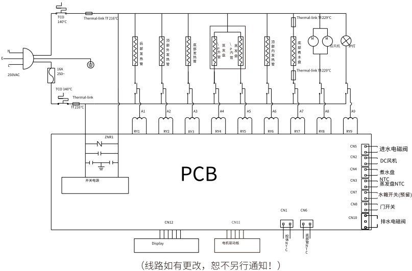
电气原理图
